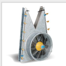
VENTOLA LINEARE PER FILARI Ø 400 MM (SUPVLN400)
