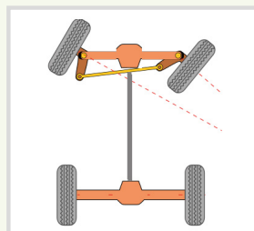
RAGGIO DI STERZATA 250 cm
